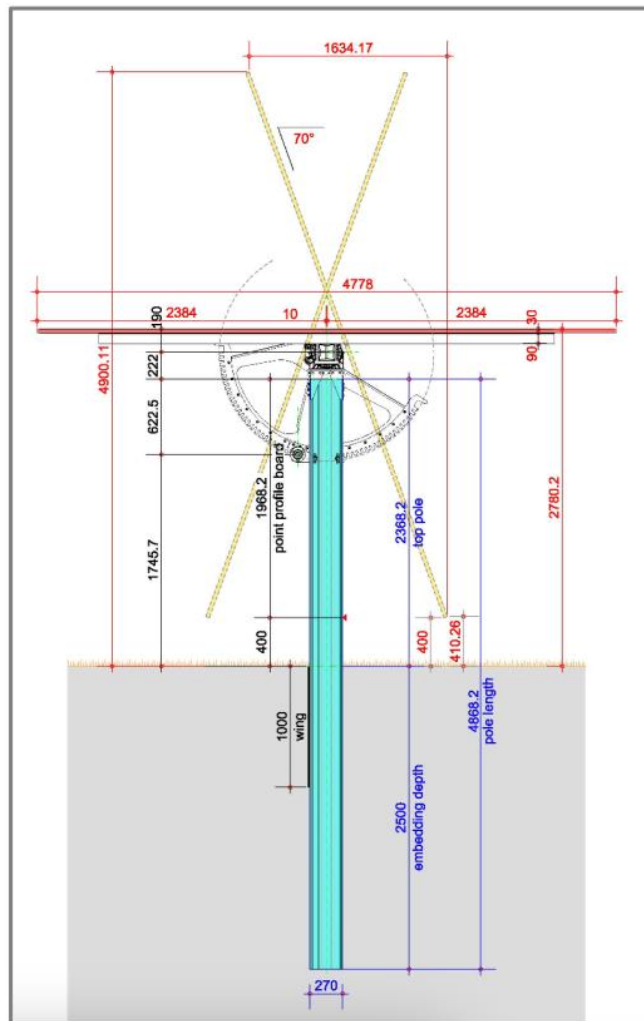
Abbildung 3: Schematische Darstellung der PV-Anlage mit Bemaßung
