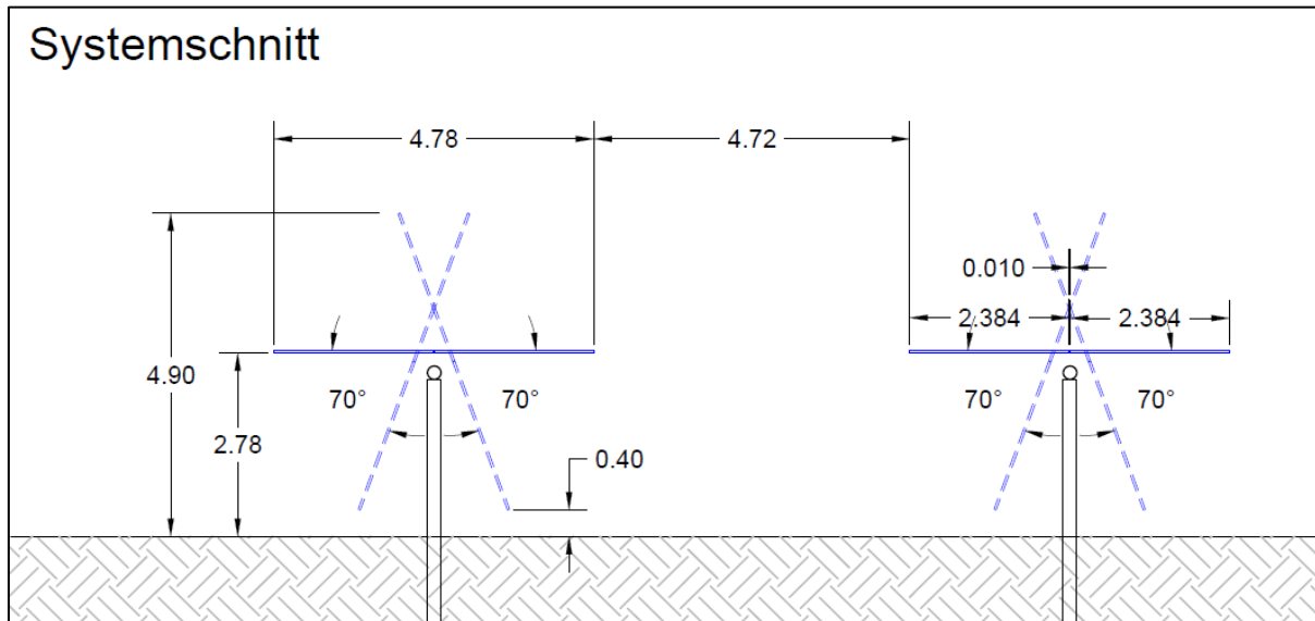
Abbildung 1: Systemschnitt mit Reihenabstand 9,50 m, Modulbelegungsplan; Mai 2024
