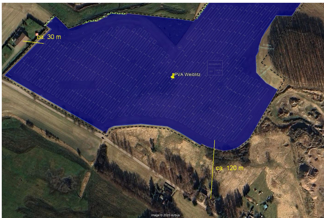
Bild 3.1: PV Fläche und die Umgebung (Quelle: Google Earth / SolPEG)
