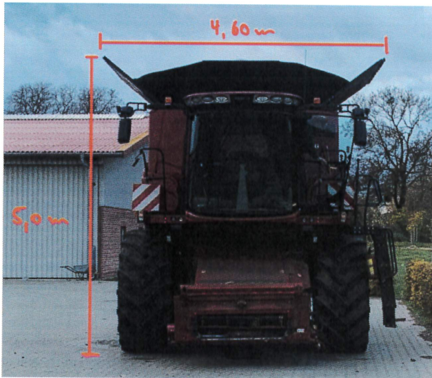
Außenmaße des Mähdreschers Case 7250.
