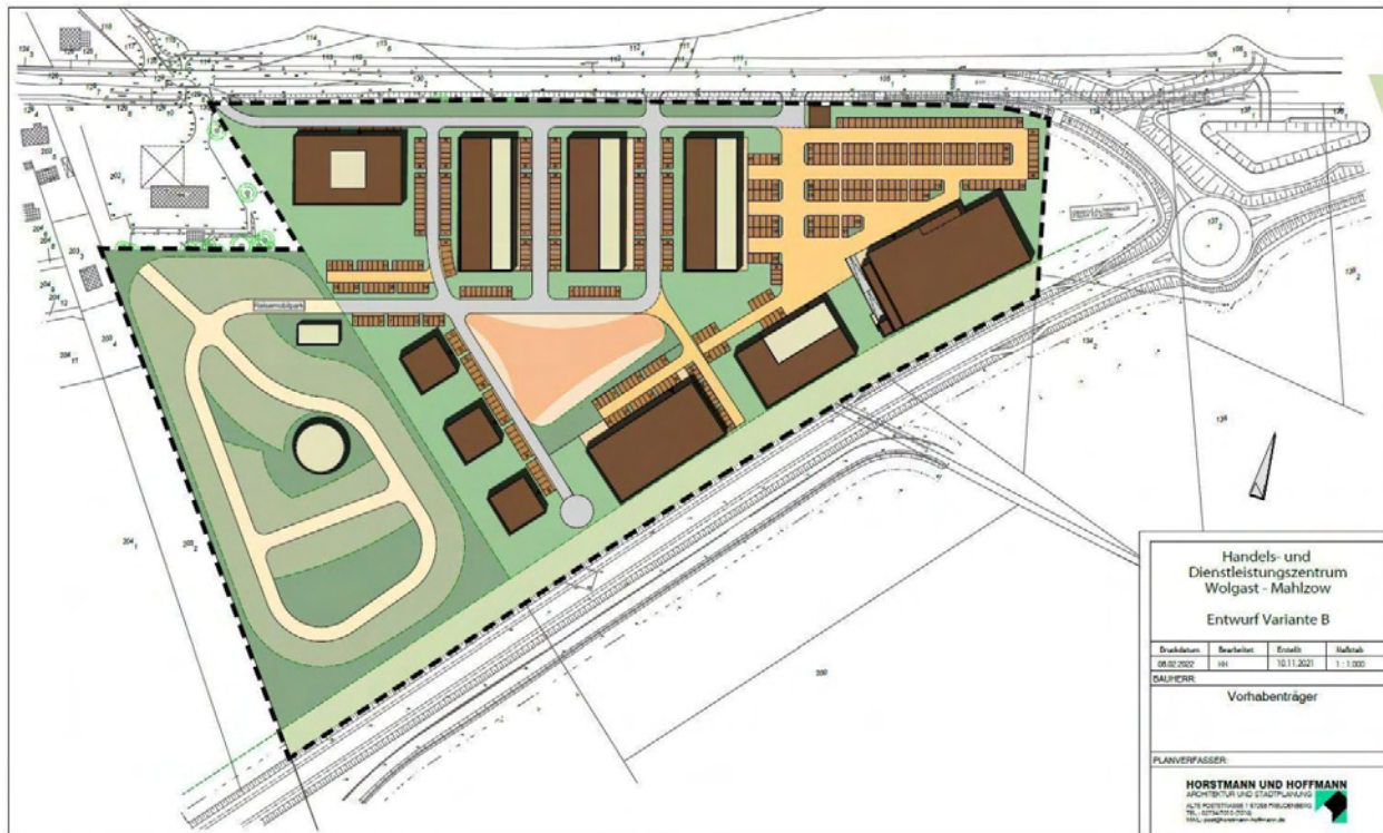
Abbildung 2: Entwurf der Variante B des Handels- und Dienstleistungszentrums Wolgast-Malzow
